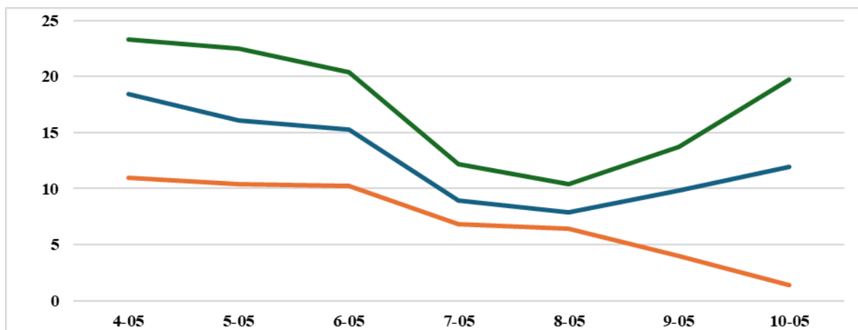
Wieża: Temperatura powietrza [°C] — T200sr — T200min — T200max
