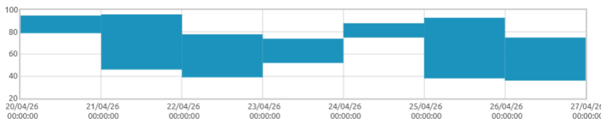
■ Małuszyn: Amplitudy wilgotności [%]
