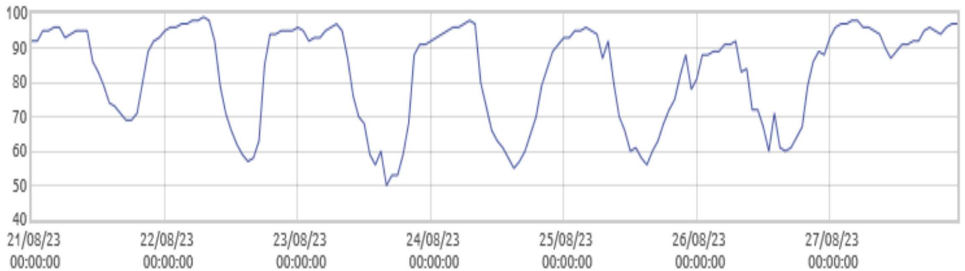
■ Swinobród: Wilgotność względna powietrza [%]
