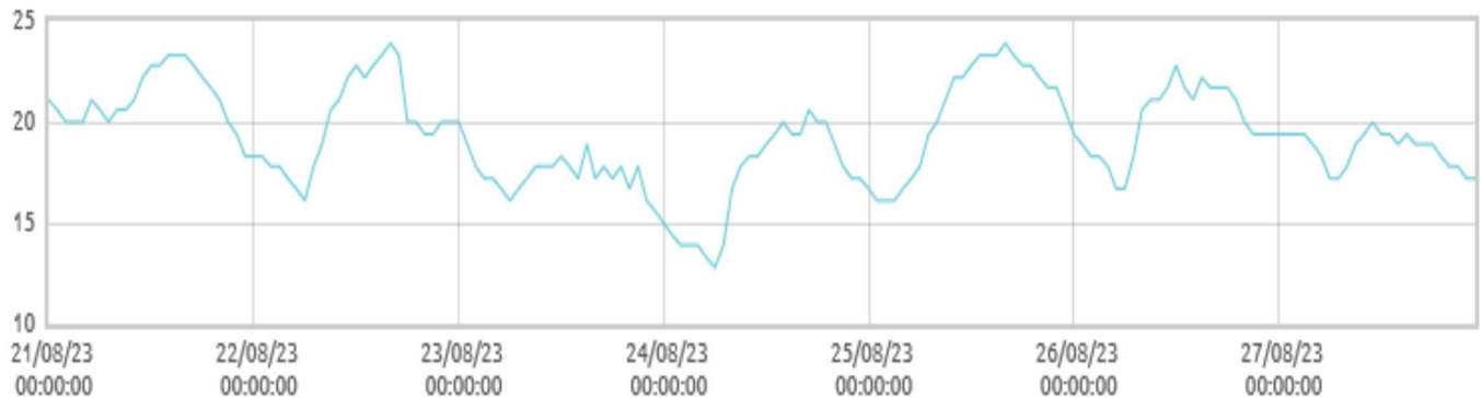
■ Świnobród: Punkt rosy [C]
