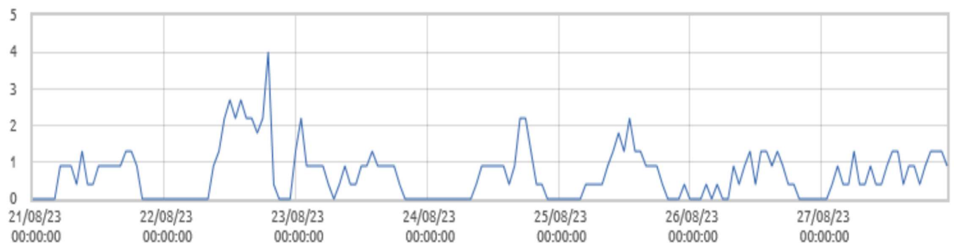
■ Swinobród: Prędkość wiatru [m/s]
