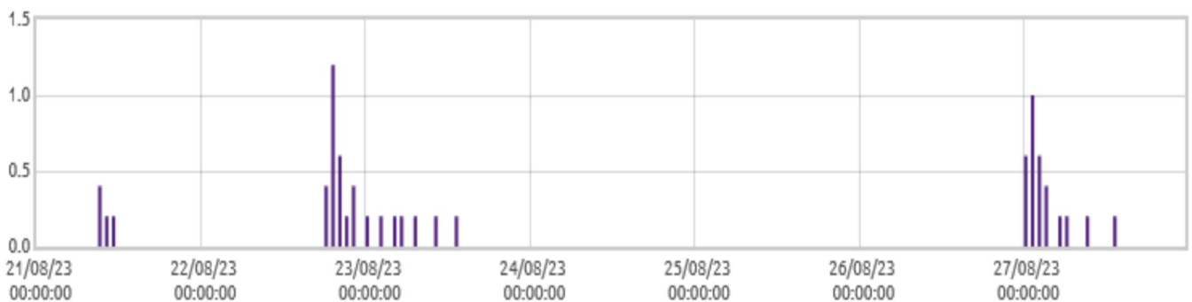
■ Świnobród: Opady deszczu [mm]
